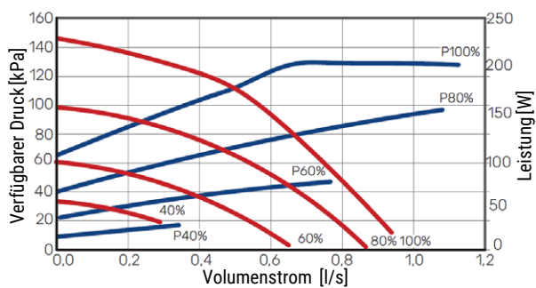
Subrox 13 C Wärmequelle
