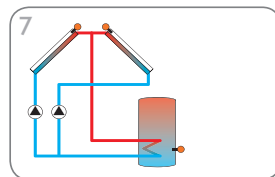
Solarsystem mit Ost-/Westdach (Seite 14)
