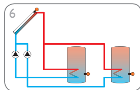
Solarsystem mit 2 Speichern, und Pumpenlogik (Seite 13)
