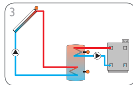
Solarsystem mit 1 Speicher und Nachheizung (Seite 10)
