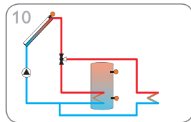
Solarsystem mit 1 Speicher und Überwärmeabfuhr (Seite 17)
