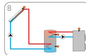
Solarsystem mit 1 Speicher und Festbrennstoffkessel (Seite 15)
