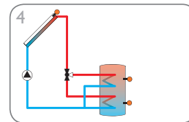
Solarsystem mit 1 Speicher und 3-Wege-Ventil zur Speicherschichtladung (Seite 11)
