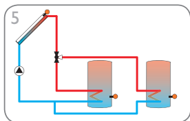
Solarsystem mit 2 Speichern und Ventillogik (Seite 12)
