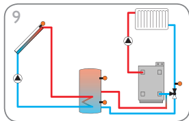
Solarsystem mit 1 Speicher und Rücklaufanhebung (Seite 16)
