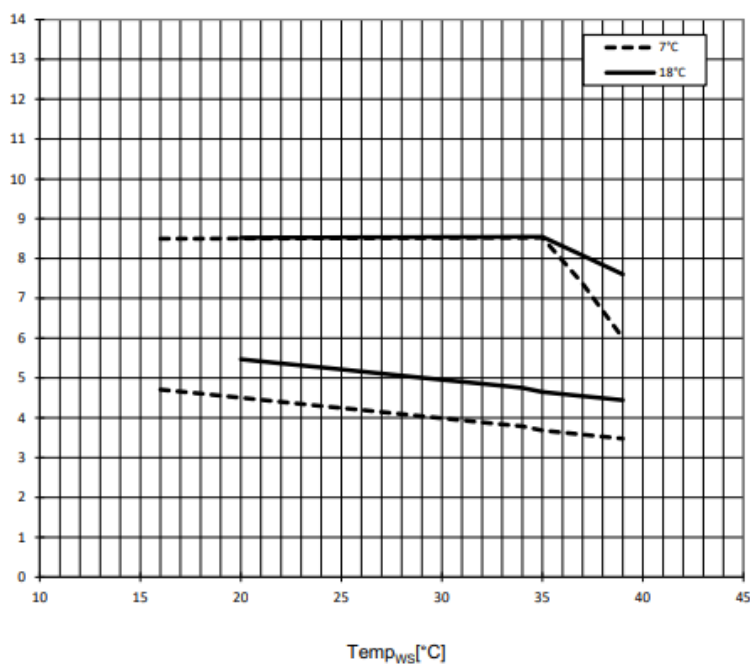
Δpmax [bar]
