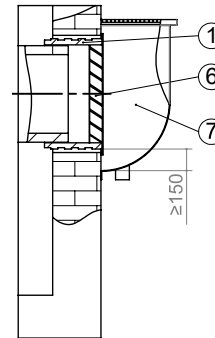
Installation d'un puits de lumière
