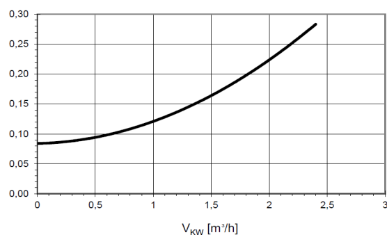
Δpmax [bar]
