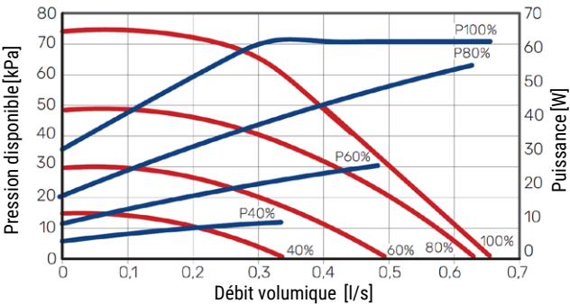
Côté chauffage
