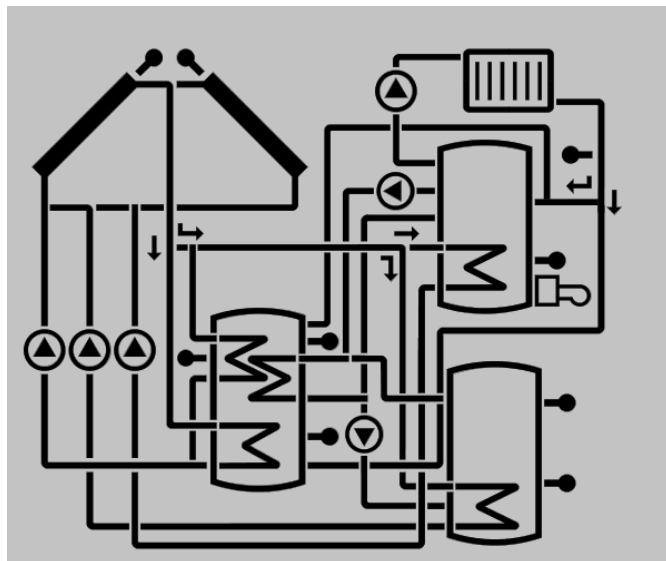
Capteurs avec sonde capteur
