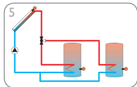
Système de chauffage solaire avec 2 réservoirs et logique de vanne (page 12)
