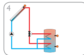
Système de chauffage solaire avec 1 réservoir et 1 vanne à 3 voies pour la charge stratifiée du réservoir (page 11)
