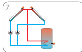
Système de chauffage solaire avec capteurs est/ouest (page 14)
