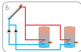
Système de chauffage solaire avec 2 réservoirs et logique de pompe (page 13)
