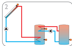
Système de chauffage solaire avec 2 réservoirs et échange de chaleur (page 9)
