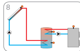
Système de chauffage solaire avec 1 réservoir et 1 chaudière à combustible solide (page 15)
