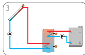
Système de chauffage solaire avec 1 réservoir et chauffage d'appoint (page 10)
