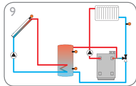
Système de chauffage solaire avec 1 réservoir et augmentation du retour (page 16)
