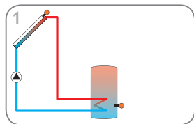
Système de chauffage solaire avec 1 réservoir (page 8)
