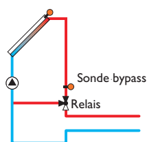
Variante vanne:
