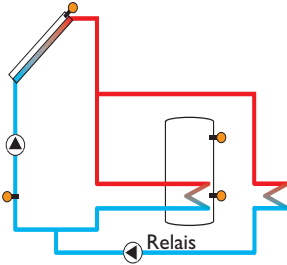
Variante pompe
