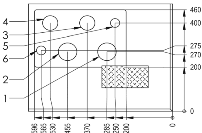
Detail Y
