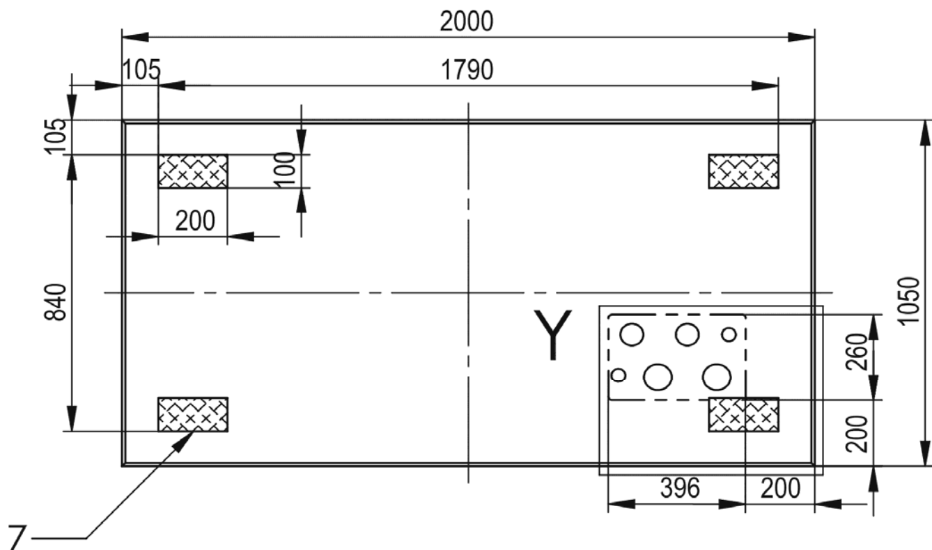
Detail Y
