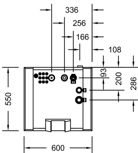
Vista dall'alto
