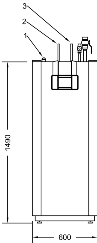
Vista anteriore
