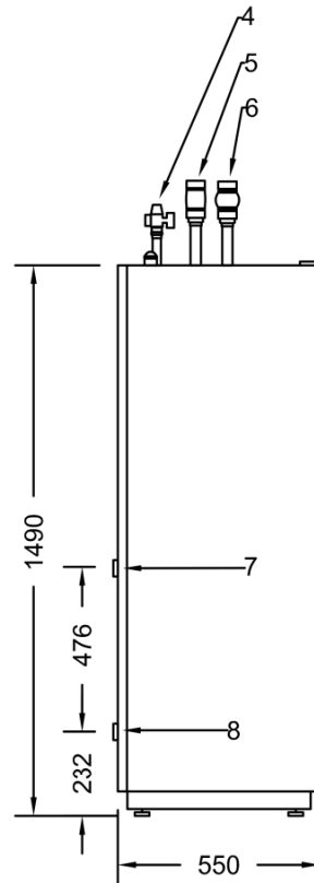
Vista laterale
