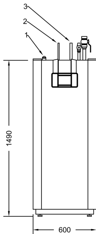
Vista anteriore
