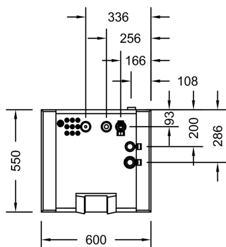
Vista dall'alto
