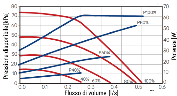
Lato riscaldamento
