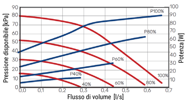
Subrox 13 C Fonte di calore
