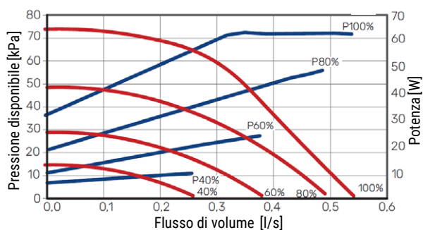
Lato riscaldamento
