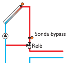
Variante valvola:
